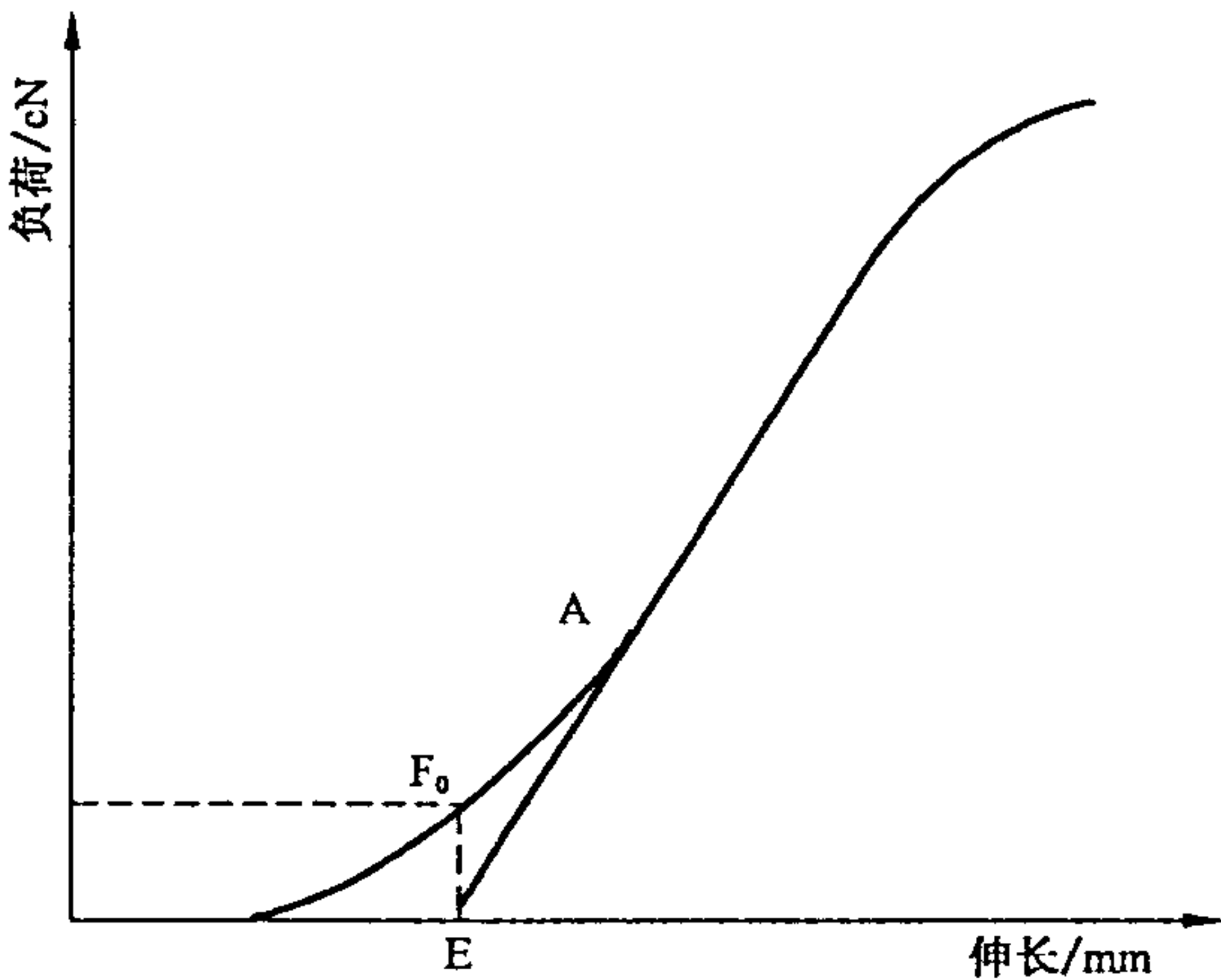
图 B.1 负荷-伸长曲线
